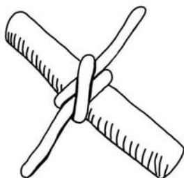
Lodní uzel
