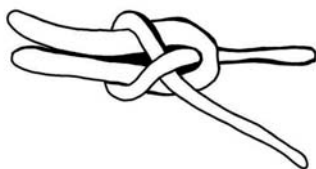
Škotová spojka
